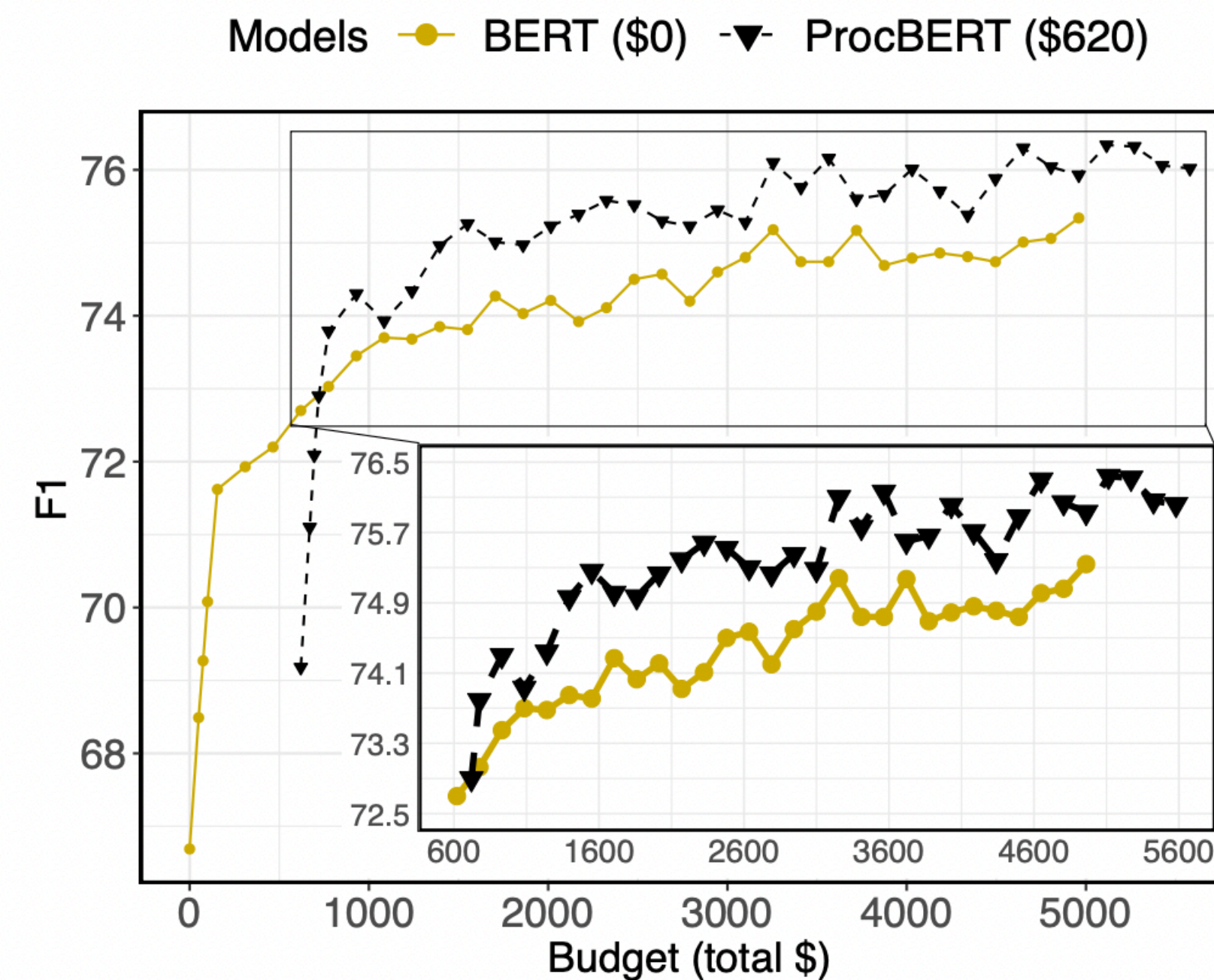
(b) CHEMSYN \Rightarrow WLP
